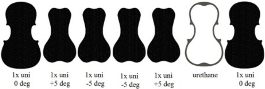
Fig. 5.13 Layup 4
