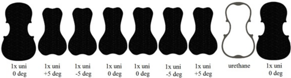
Fig. 5.12 Layup 3
