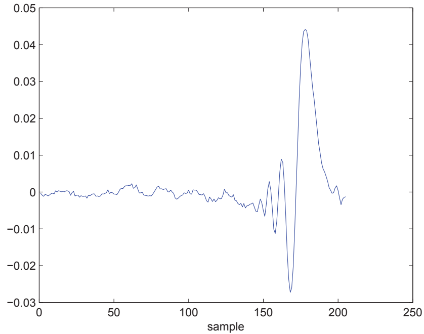
Fig. 4.10 \tilde{a}_{exc}(n)
