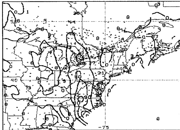
a) 15-16 Oct 1954
