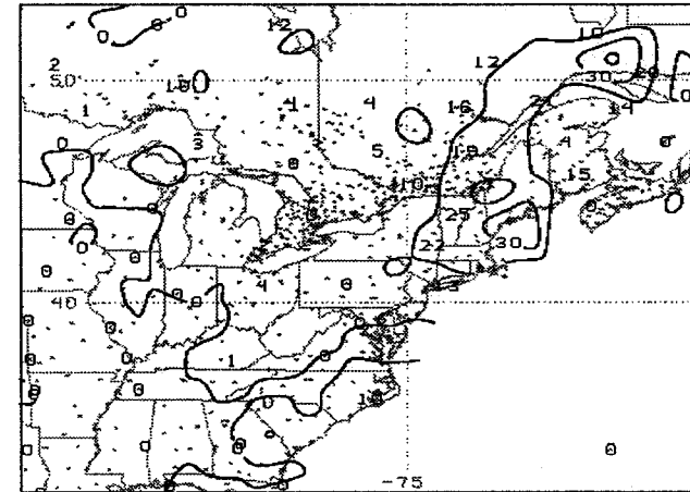
b) 5 Sept 1985
