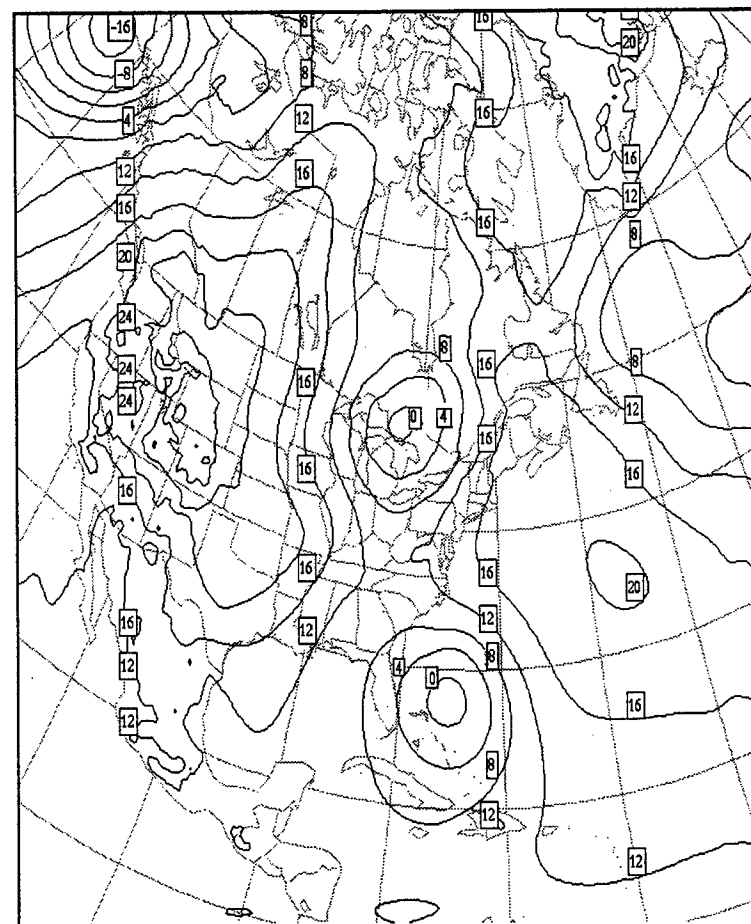
b) 03 UTC 15 Oct
