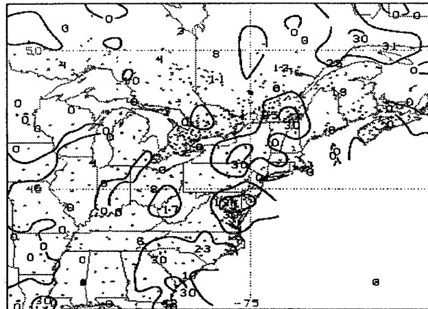
c) 14-15 Oct 1995
