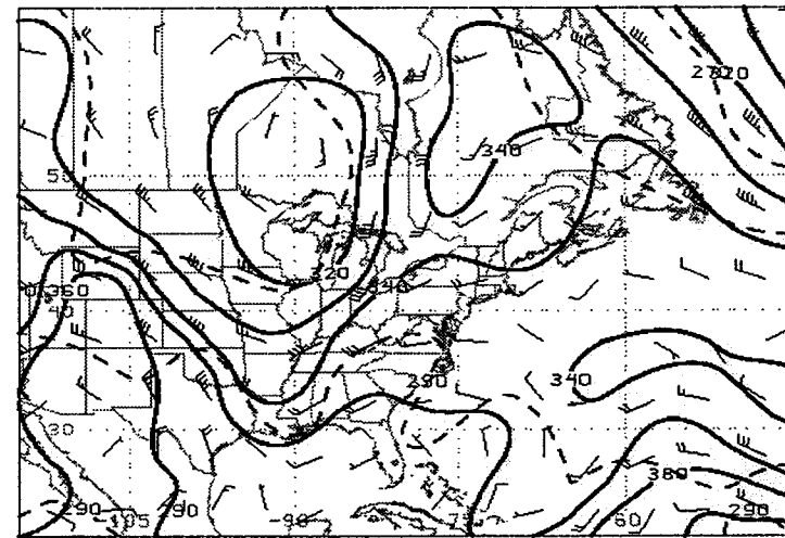
h) 12 UTC 09 Sept 1999
