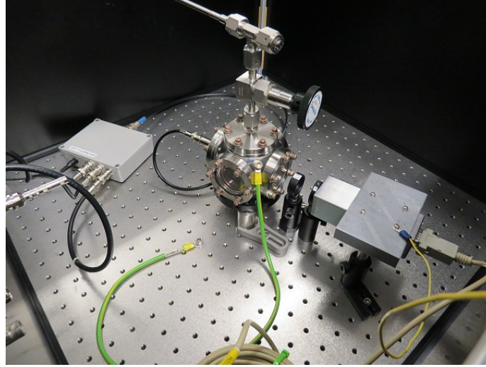
(a) CSP, ELS Chamber and Flash Lamp in Dark Box.
