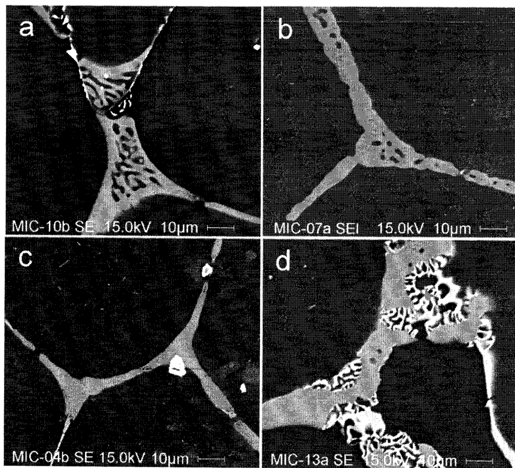
Figure 4-10 -BSE images of MgCeIn alloys with approximately 0.27at%Ce: (a) 0.00at%In, 0.22at%Ce (b) 0.22at%In, 0.27at%Ce (c) 0.44at%In, 0.28at%Ce (d) 0.64at%In, 0.26at%Ce.
