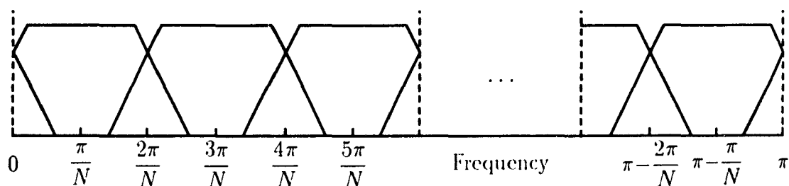
(d) Filter responses for system T2
