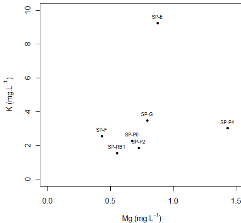
Figure 3.4. (Continued). c/ Mg vs. K.
