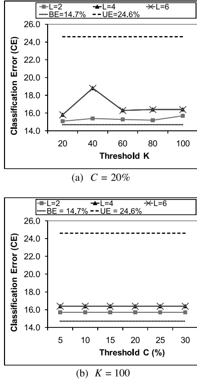
Fig. 6. Adult dataset.
